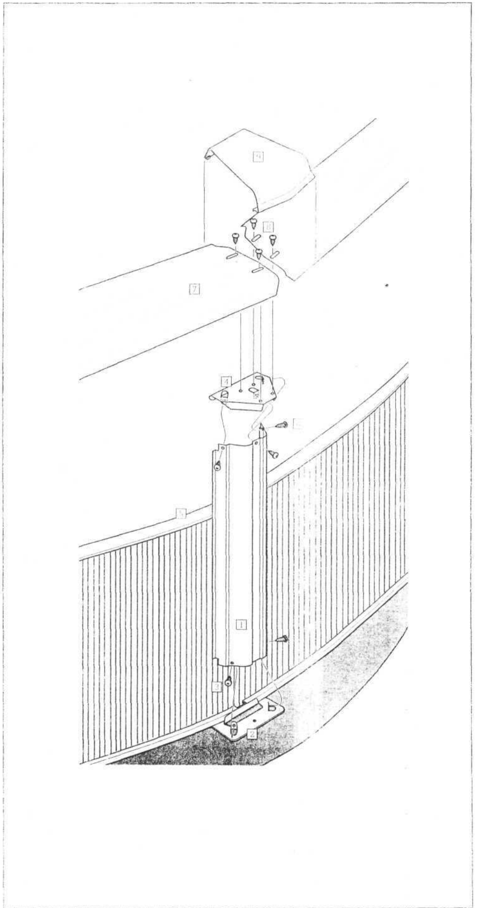
Схема крепления вертикальной стойки, верхней рейки и верхнего соединителя
